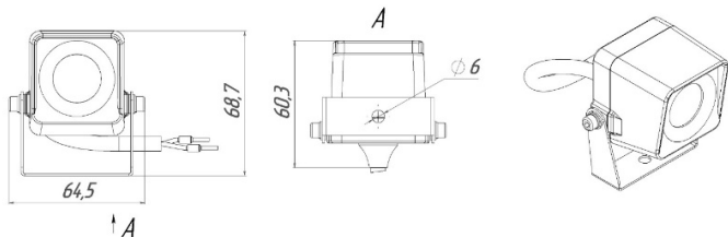
Рисунок 1 Светильник «L-mouse»
